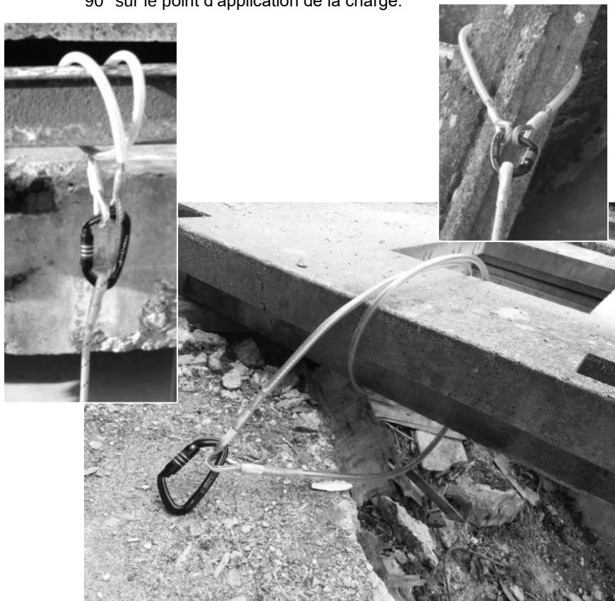
Illustration 22 : amarrages avec élingue en acier
