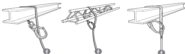
Illustration 26 : ceinture d'un ancrage
