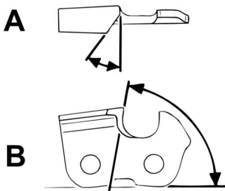
Illustration 46 : angles d'affutage
