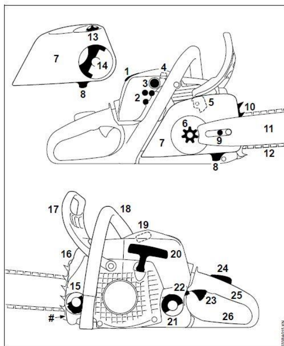
Illustration 1 : les parties de la tronçonneuse
